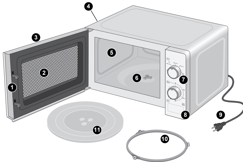
Рис. 1: Компоненты прибора
