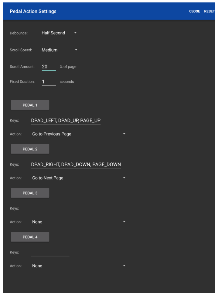
Abbildung 62 - Pedal Aktionseinstellungen
