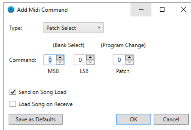
Abbildung 72 - Der MIDI-Befehlsdialog
