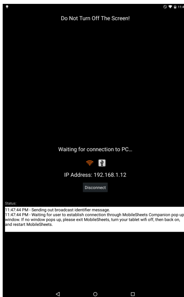
Abbildung 65 – Der Sync-Bildschirm
