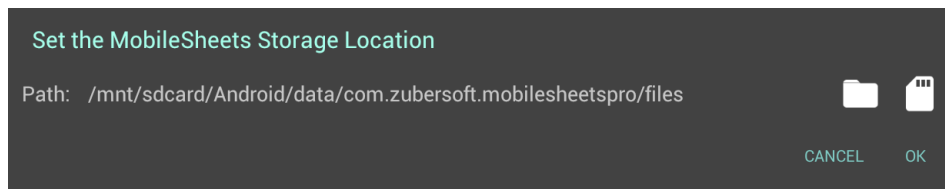
Abbildung 11 – Die Datenspeicherung
