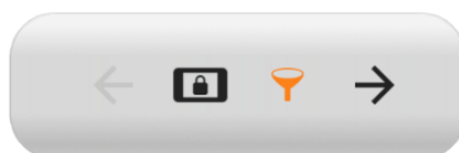
Abbildung 4 – Schwimmende Symbolleiste
