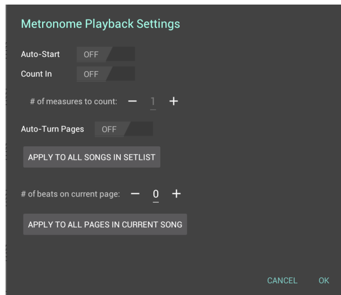
Abbildung 45 – Metronom-Wiedergabeeinstellungen
