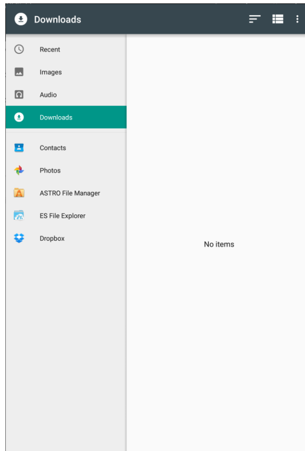
Abbildung 14 – Google-Dateiauswahl
