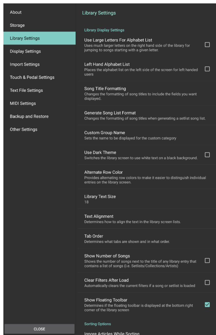
Abbildung 64 – Der Einstellungsbildschirm
