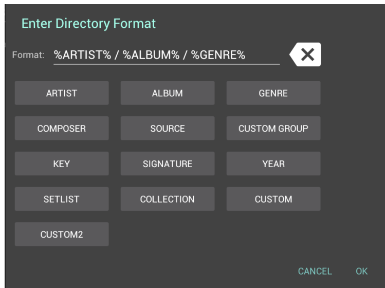
Abbildung 16 – Dialogfenster Meta-Daten
