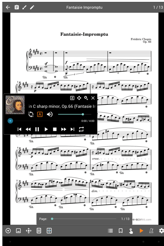
Abbildung 32 – Die Liedüberlagerung
